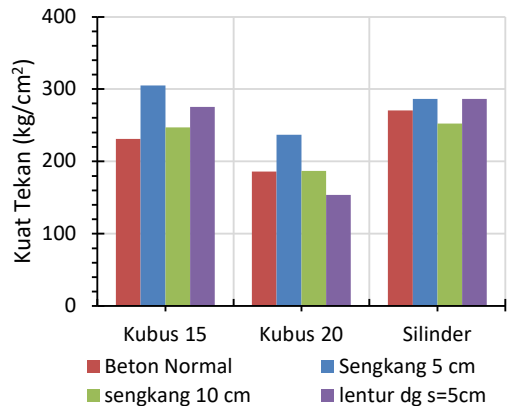
Gambar 7 Grafik Kuat Tekan dan Benda Uji Dari grafik di atas, dapat diketahui bahwa benda uji dengan penulangan lentur dan pengekanan mampu meningkatkan kuat tekan beton pada berbagai bentuk benda uji, baik kubus maupun silinder. Benda uji kubus cenderung memiliki kuat tekan lebih tinggi karena distribusi tekanan lebih terpusat di area tertentu, ditambah dengan efek pengekanan internal alami dari bentuknya. Sementara itu, benda uji silinder lebih
