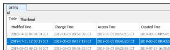
Gambar 7 Waktu upload file dan penghapusan
